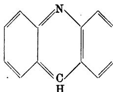
Acridin.
